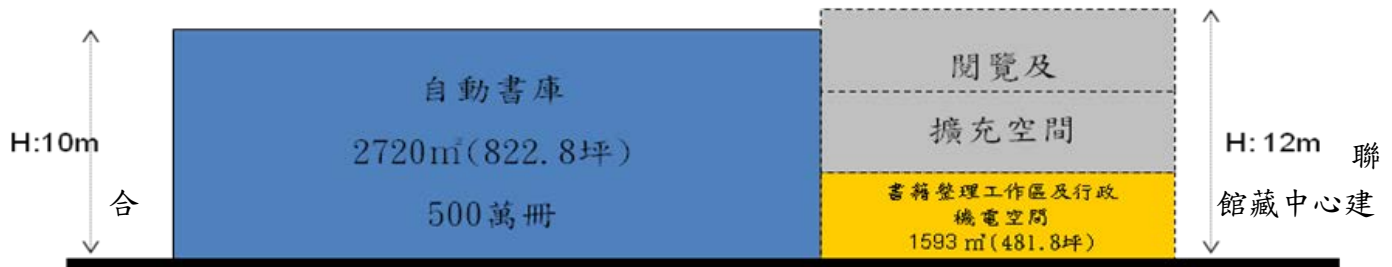
築構成方案剖面示意圖
